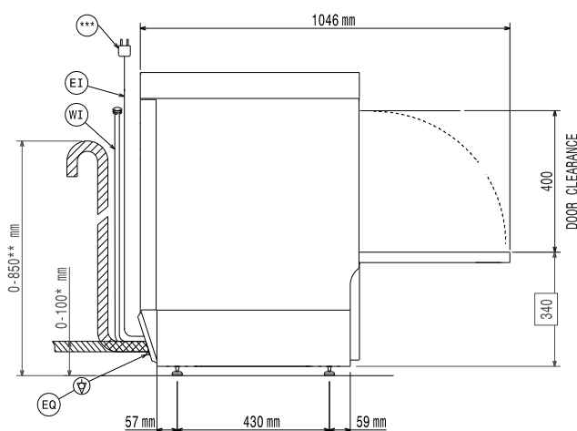
Zij aanzicht
